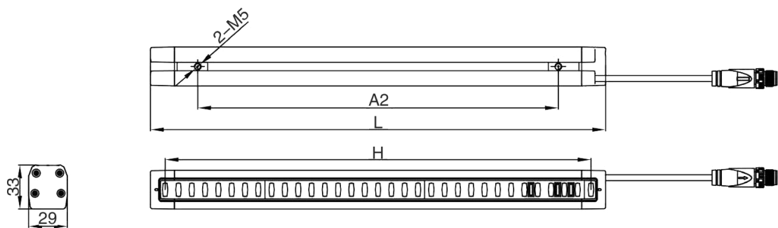
B（背部滑块）安装方式
